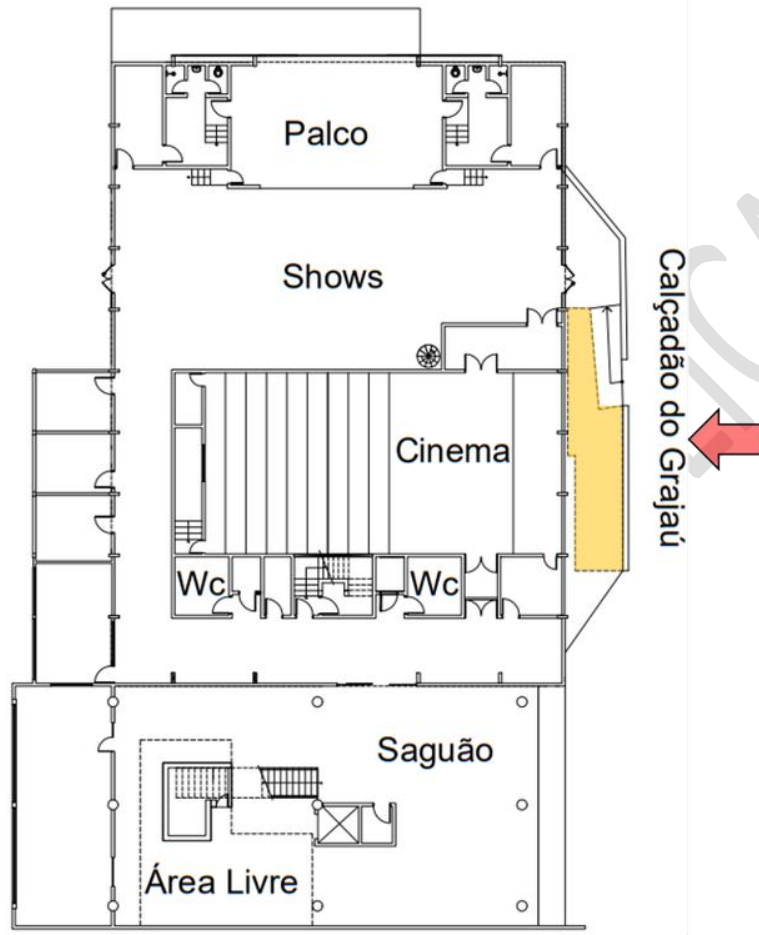
Figura 10 – Planta Baixa: Térreo
