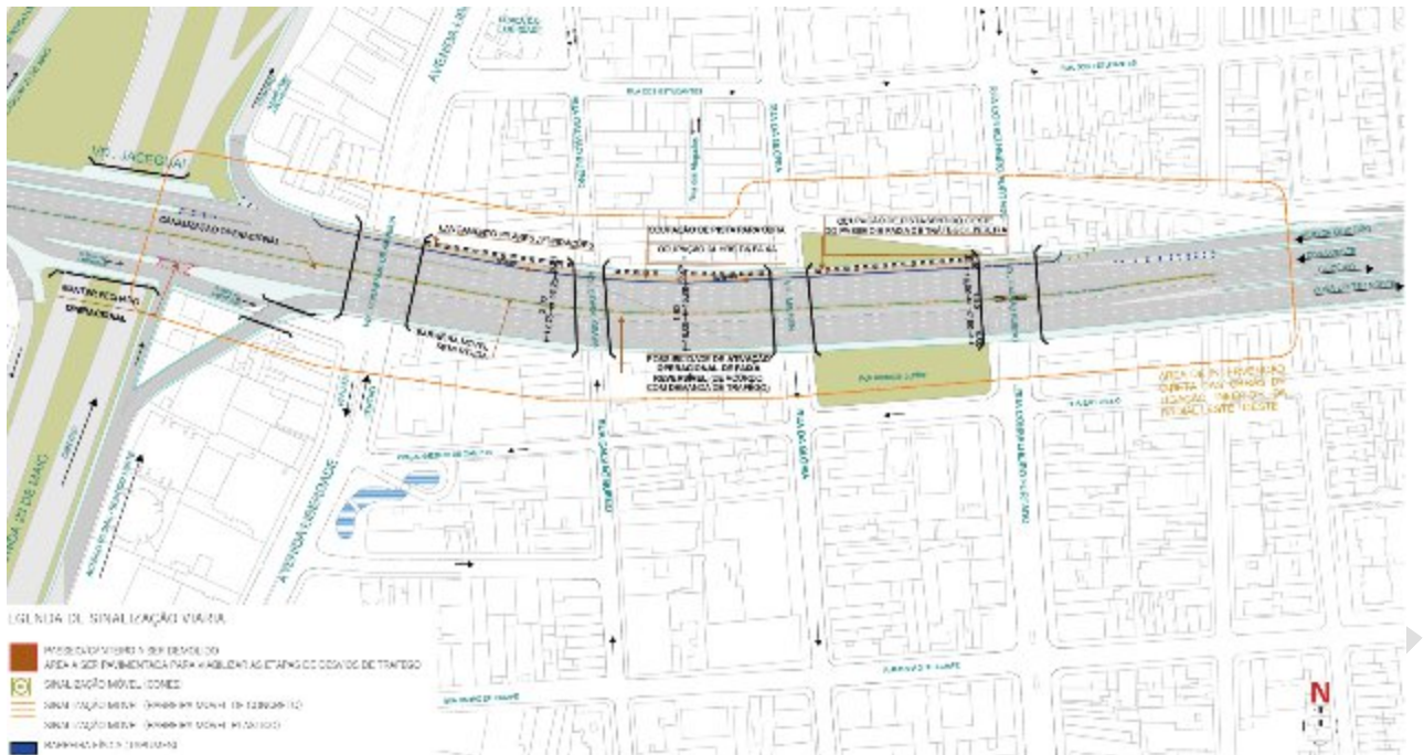
Figura 46 - Interrupções e sinalizações durante a implantação das fundações e pilares da extremidade norte
