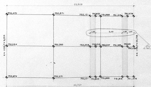
PLANTA - LAJE TETO ESC. 1/100
