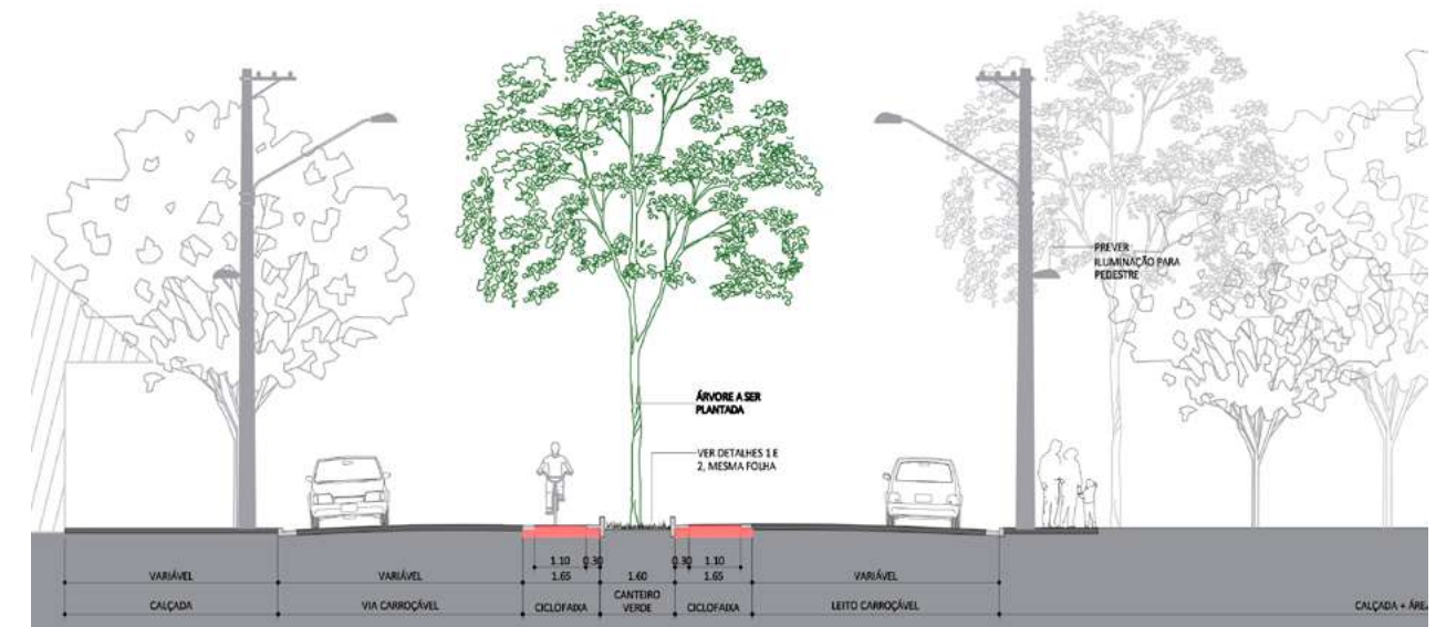
Fig. 29 - Corte do Corredor Verde Benjamin Mansur integrado ao projeto de ciclofaixa
