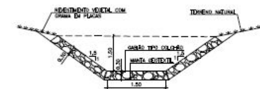
DETALHE DE REVESTIMENTO DE CANAIS DE ESCOAMENTO COM GABIÕES TIPO MANTA b=1,50m : h=1,50m S/ESCALA
