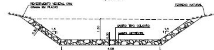
DETALHE DE REVESTIMENTO DE CANAIS DE ESCOAMENTO COM GABIÕES TIPO MANTA b=4,00m : h=1,50m S/ESCALA
