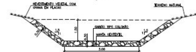
DETALHE DE REVESTIMENTO DE CANAIS DE ESCOAMENTO COM GABIÕES TIPO MANTA b=3,00m : h=1,50m S/ESCALA
