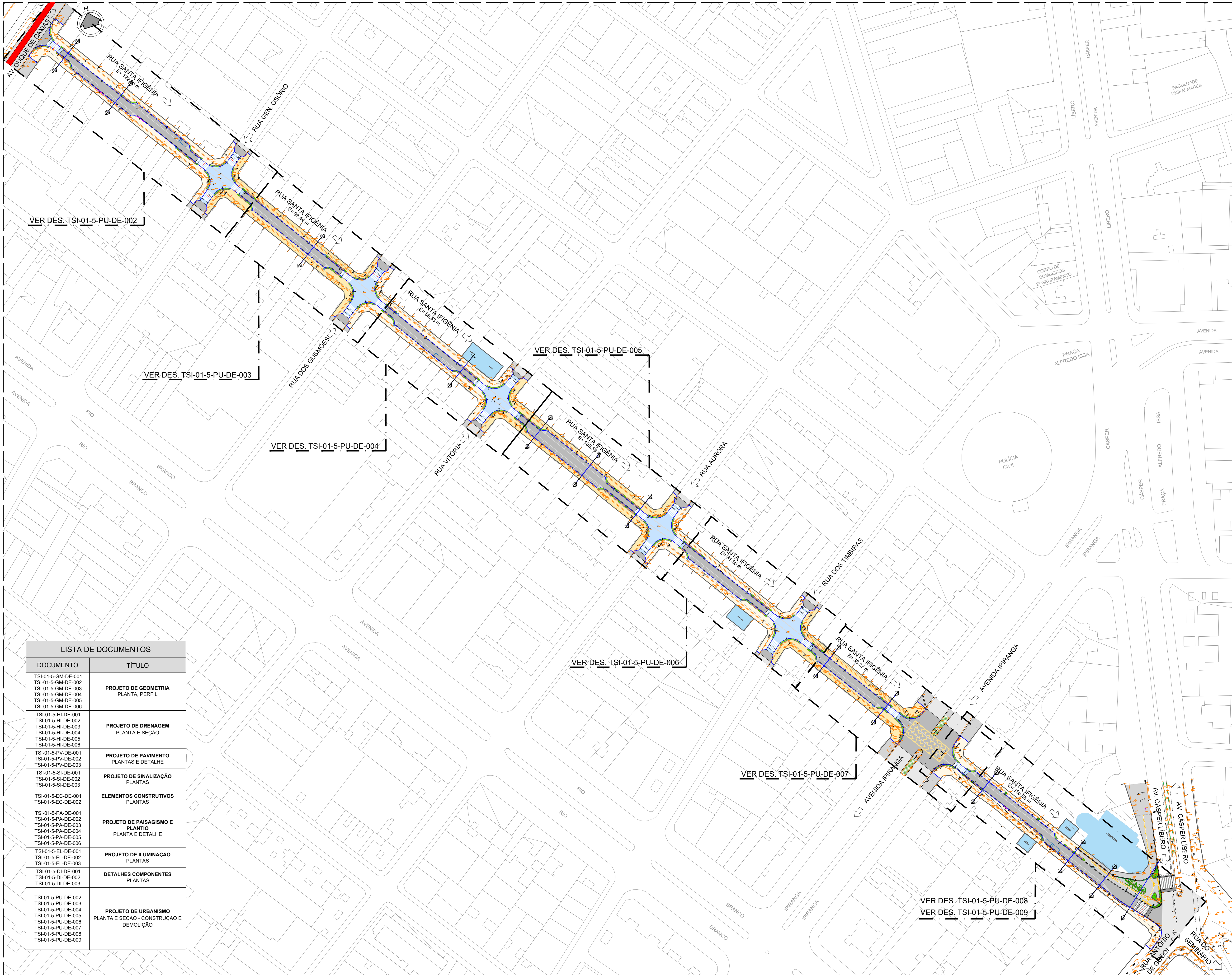
PLANTA DE IMPLANTAÇÃO 1:1000
